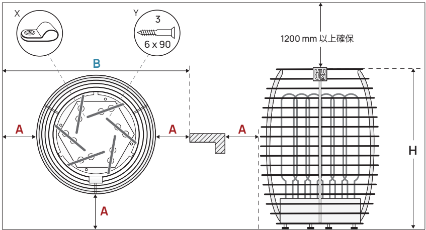
図1 サウナヒーターの設置位置
